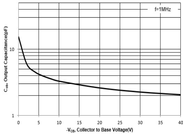
Fig. 6 Output Capacitance
